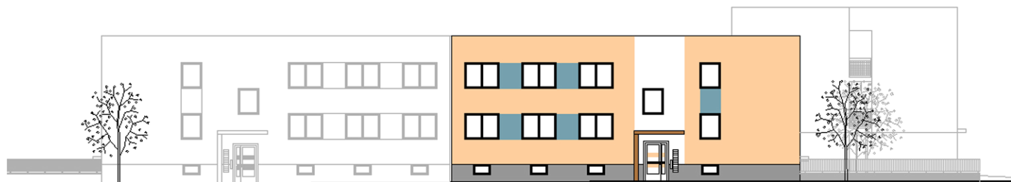
POHLED ZÁPADNÍ Z OBSLUŽNÉ KOMUNIKACE NA ULICI HOROVA
